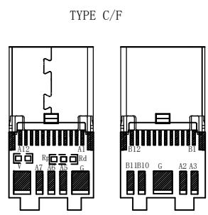
TYPE C3.0 母头焊接面
