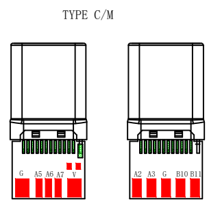
TYPE C3.0 公头焊接面
